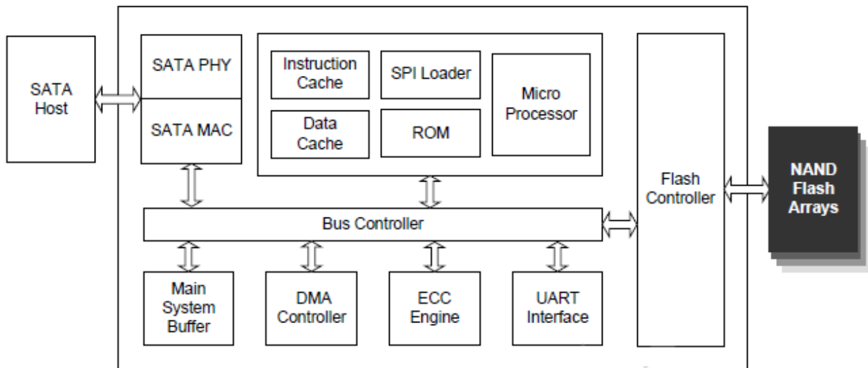
Figure 2: Innodisk mSATA mini 3ME2 Block Diagram
