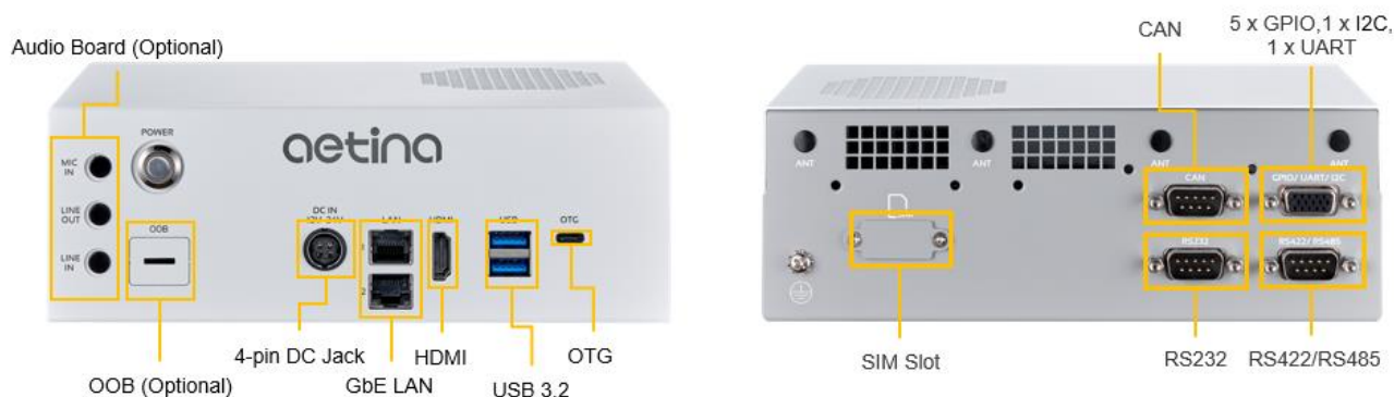
Figure 2.1 AIE-KO22/AIE-KO32/AIE-KN32/AIE-KN42 I/O Interface
