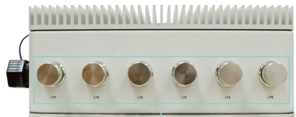
Antenna (2 WiFi & 4 LTE)
