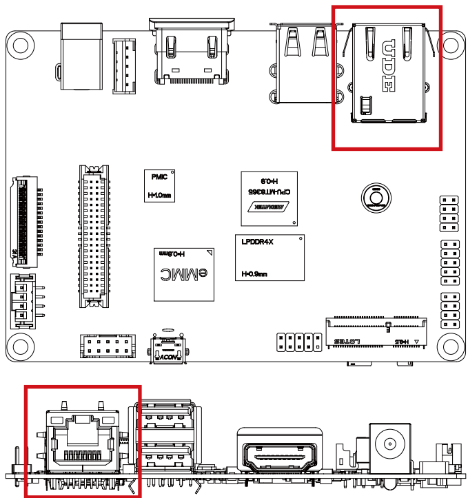
LAN Connector
