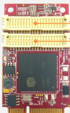
CN1(40DP-1.25), VGA X 2
